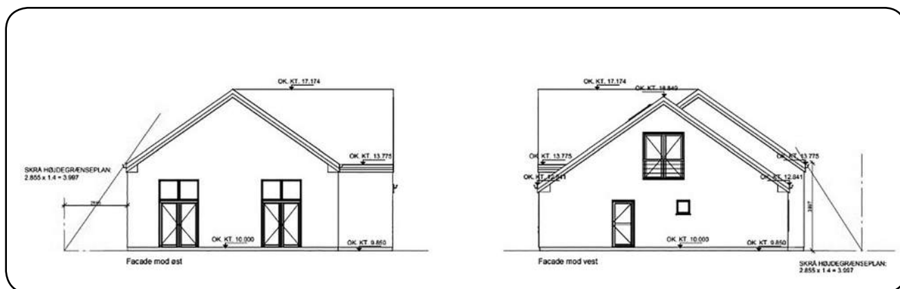
Arkitektens godkendte tegning af gavle mod øst og vest
