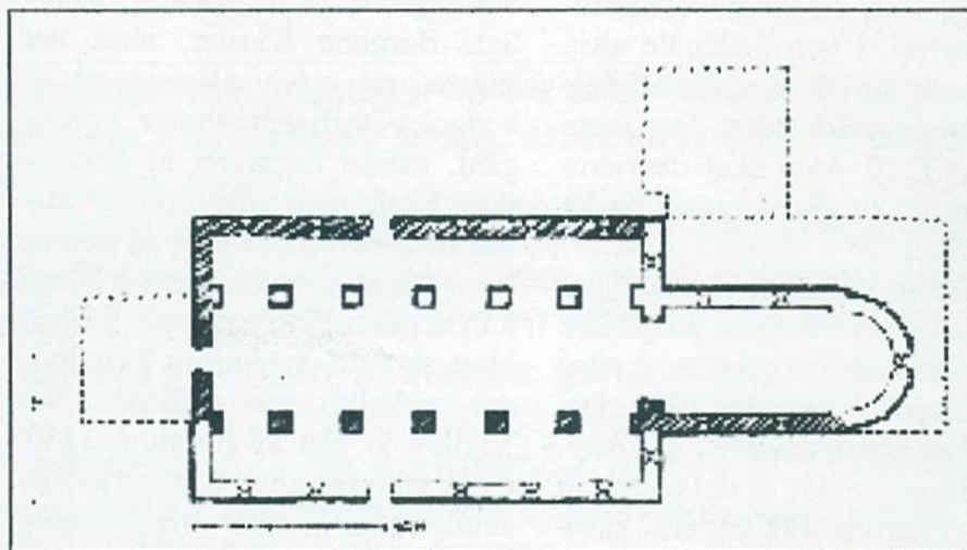
Grundplan af Vrejlev "1160-kirke" Bevaret romansk kvaderværk er skraveret. Med stiplede linie er angivet senere tilbygninger, herunder den fjernede udbygning på nordvæggen
