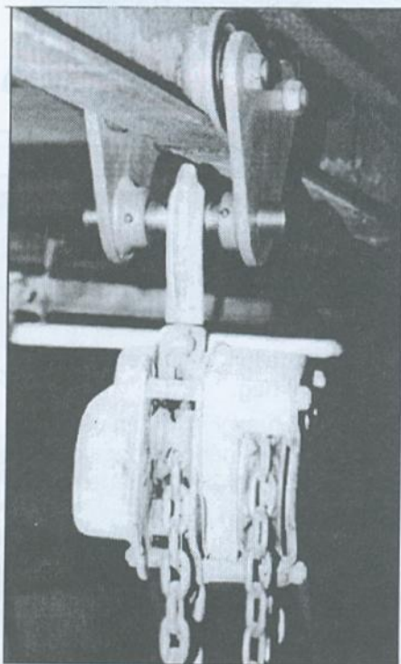
Her er en lille løbekat m talje....
